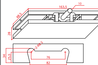
CK-020 Üst Menteşe Upper Hinge
