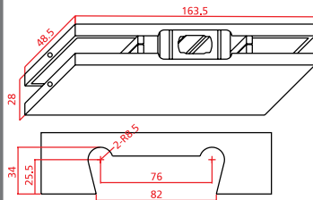
CK-010 Alt Menteşe Base Hinge
