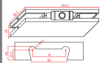
CK-030 Üst Menteşe Upper Hinge
