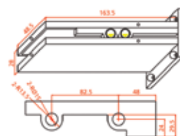
CK-050 Üst (T) Menteşe Upper (T) Hinge
